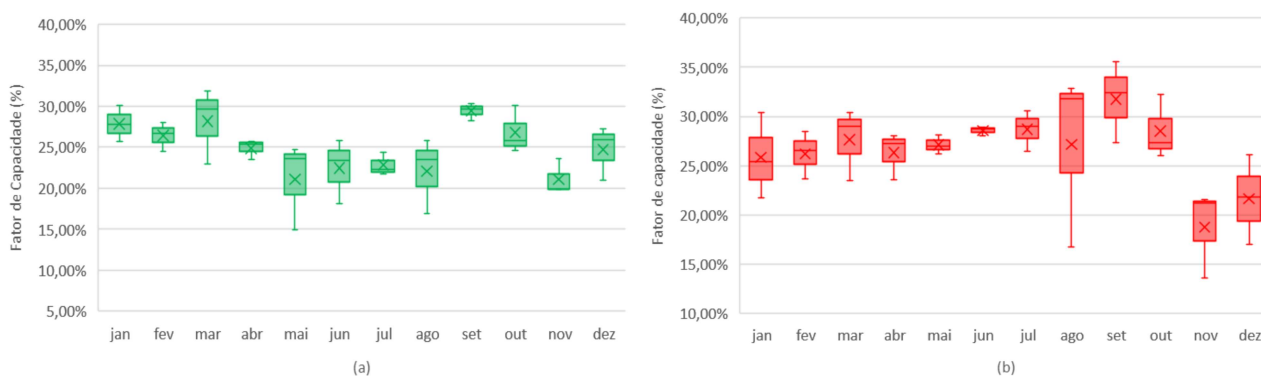
Figura 6 - Fator de capacidade médio anual. Em (a) conjunto B JL. Em (b) conjunto Sertão Solar Barreiras.
