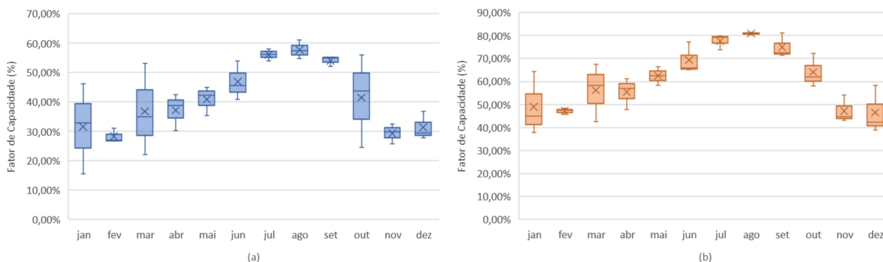
Figura 4 - Fator de capacidade média anual. Em (a) conjunto Brota de Macaúbas. Em (b) conjunto Morro do Chapéu.
