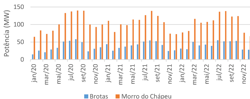
Figura 3- Potência média mensal eólica dos conjuntos eólicos para o período de 2020 a 2022.
